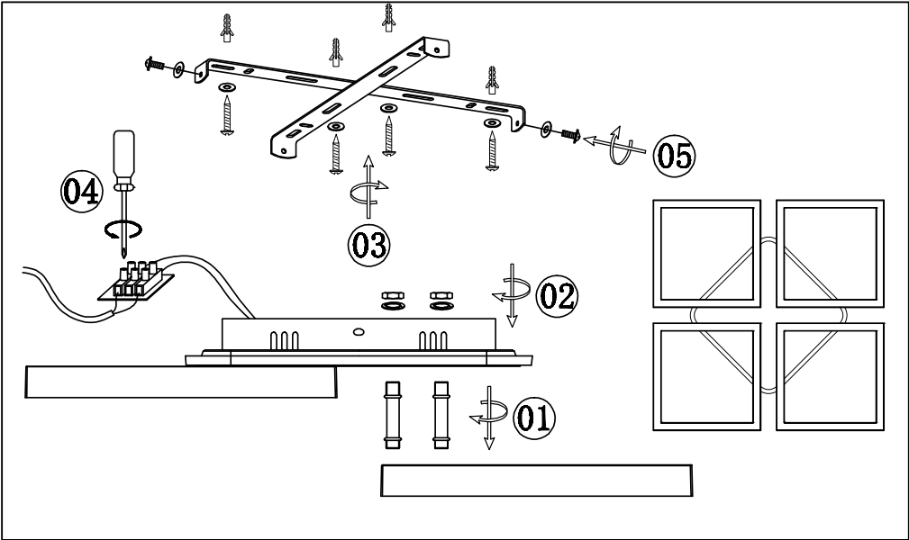
Схема інсталяції AL6490ARD / AL6490-1ARD
