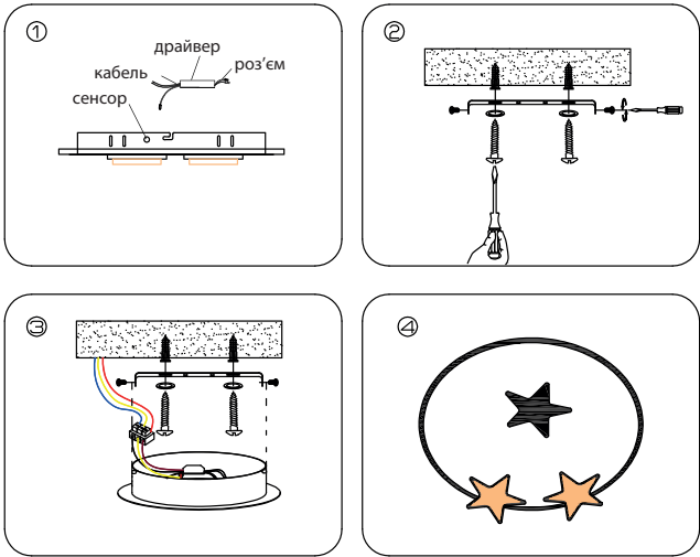
Схема інсталяції AL6104ARD
