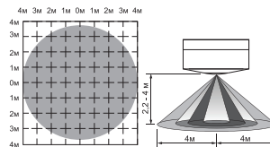
Схема зон охвата датчика ( 360^{\circ} ):
