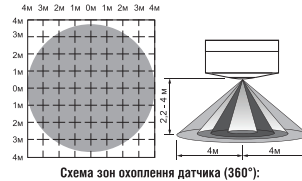
Схема зон охоплення датчика (360°):
